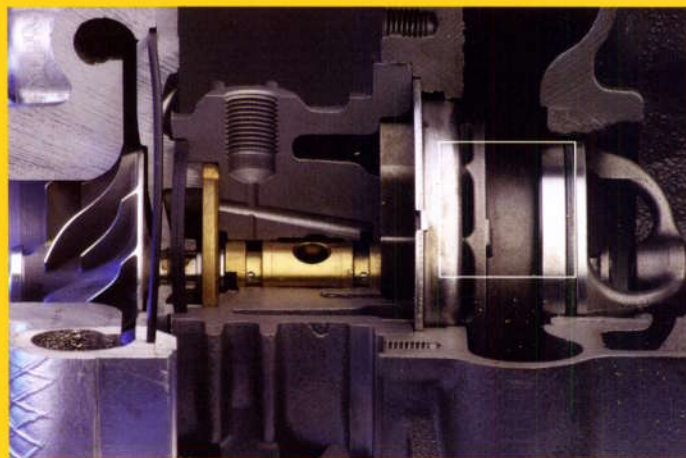
6.7 Vannes en position fermée: entraînement limité
