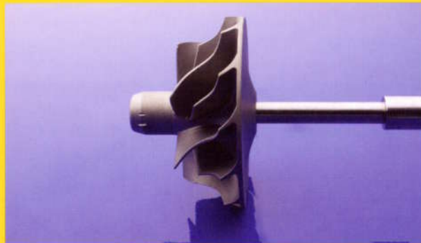
4.4 Roue de compresseur boreless superback
