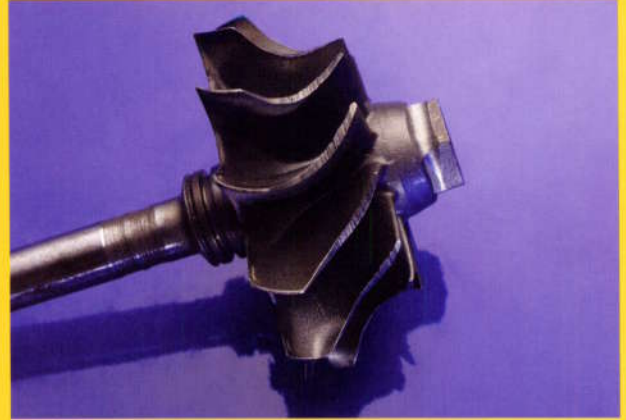
7.3 Frottement de la roue de turbine
