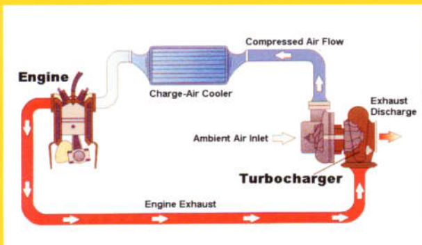
4.1 Diagramme du turbocompresseur
