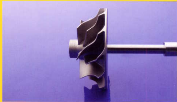
4.2 Roue de compresseur flatback
