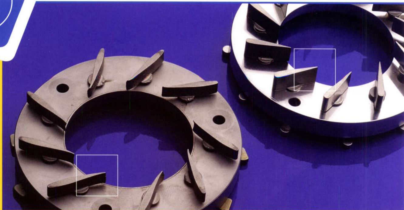
7.13 Impact d'un objet étranger sur le nozzle ring
