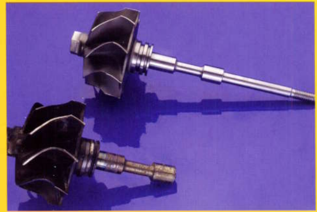
7.4 Arbre de turbine cassé
