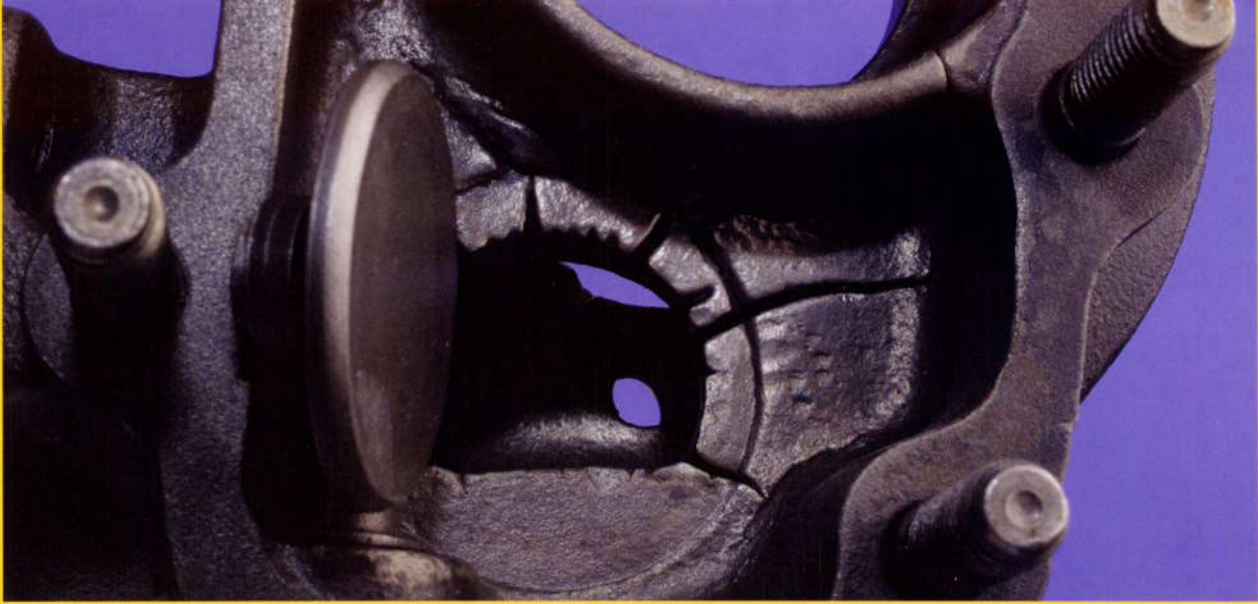
7.23 Fissures dans le carter de turbine
