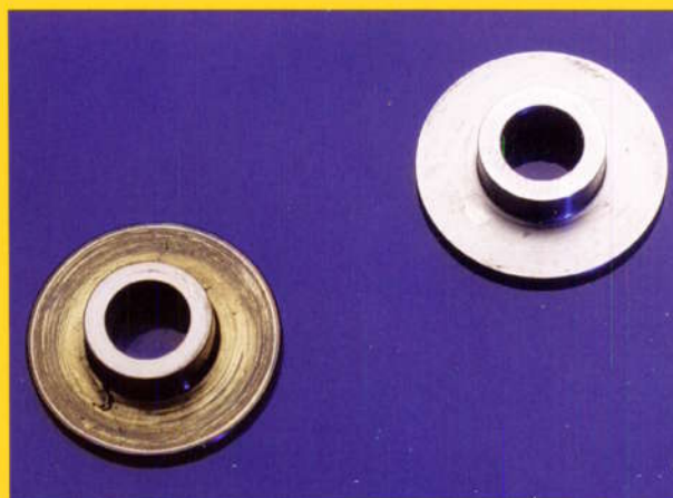
7.17 Collet de palier endommagé et nouveau collet de palier
