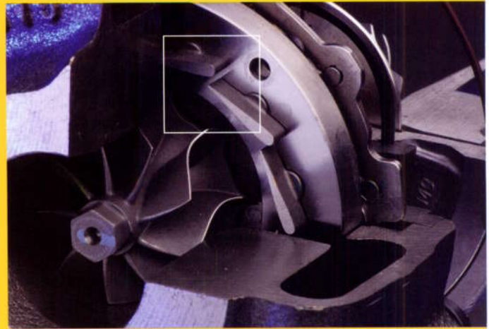
6.3 Vannes en position fermée: entraînement complet de la turbine
